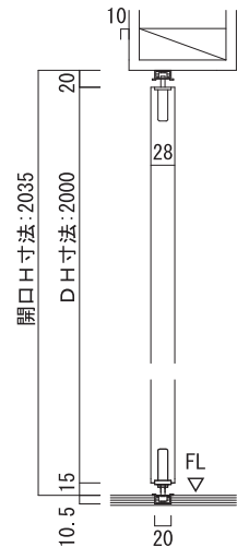
上下レール
