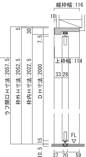
上下レール
