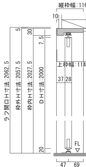
上レール
