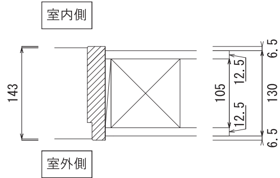
縦枠納まり
