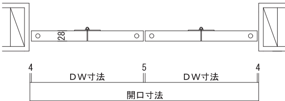
4枚扉(枠なし)
