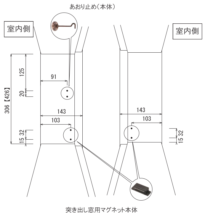
縦 枠
