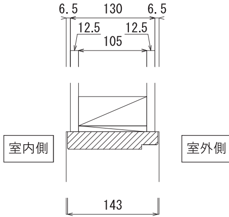
上枠納まり
