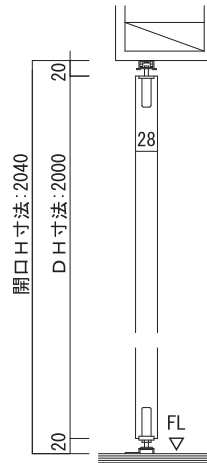
上レール
