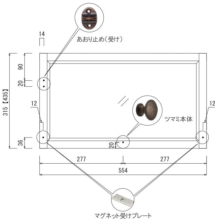
窓 (室内側)
